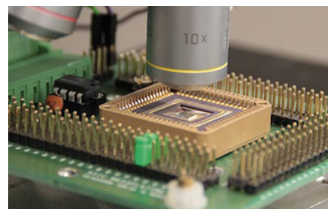
Charakterisierung eines Opto-ASICs unter dem Mikroskop
