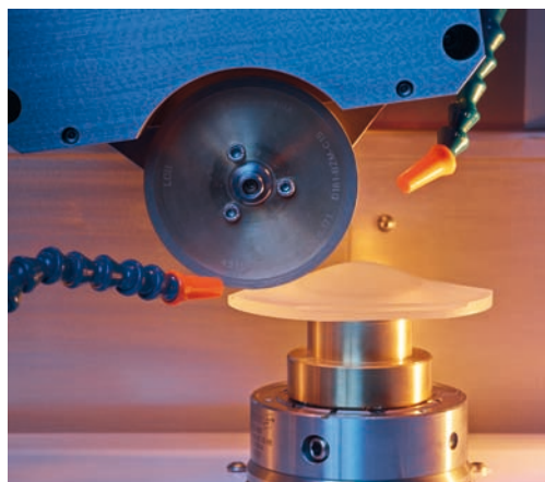
Asphäre mit formgeschliffenem Randzylinder, bearbeitet mit der Satisloh SPM-200
