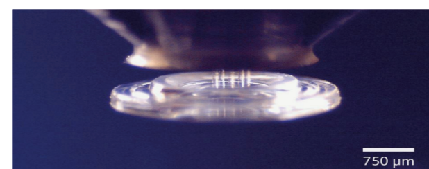
Adhäsiver Greifer zur Handhabung von Mikrolinsen Adhesive gripper for microlens handling
